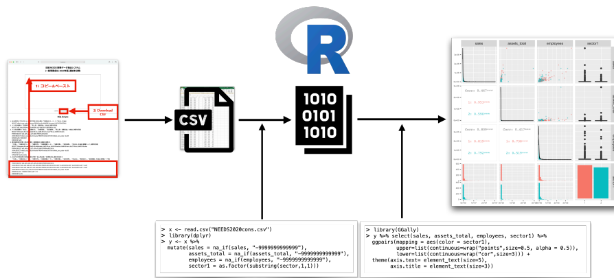
図 11: CSV ファイルとしてダウンロードされたデータファイルを R を利用して可視化する工程
