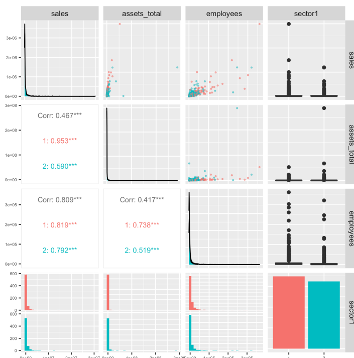
図 10: 対角ブロックには売上高 ( sales ), 資産合計 ( assets_total ), 従業員数 ( employees ) に関する推定された密度関数と、日経産業分類 ( sector1 : 大分類) の頻度が描かれている。また、上三角ブロックには、売上高 ( sales ), 資産合計 ( assets_total ), 従業員数 ( employees ) の 2 つの組合せに関する散布図と最終列には、それぞれのデータのボックスプロット (1: 製造業, 2: 非製造業) が描かれている。さらに、下三角ブロックには、売上高 ( sales ), 資産合計 ( assets_total ), 従業員数 ( employees ) の 2 つの組合せに関する相関係数が与えられており、最終行には、それぞれのデータ頻度のバーチャート (1: 製造業, 2: 非製造業) が描かれている。
