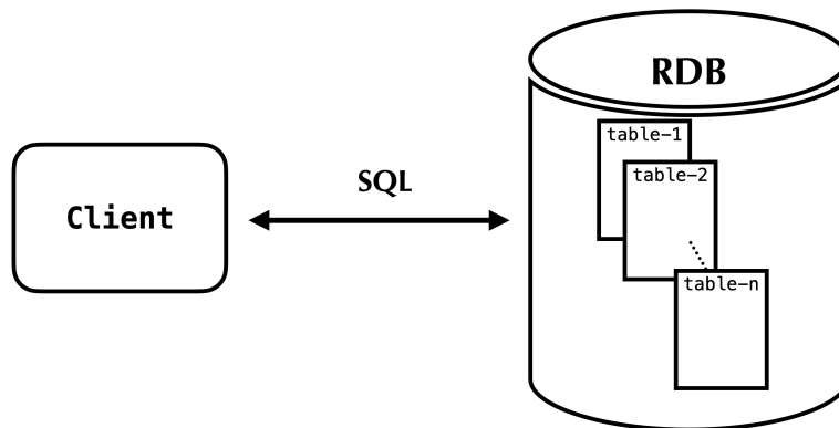
図 14: SQL の役割
