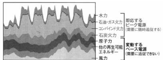
図2 スペインにおける電力系統運用
